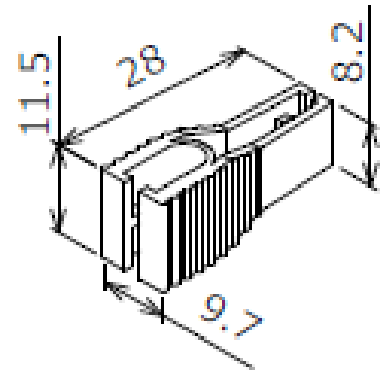
別売品 ヒューズブラー 材質：POM
