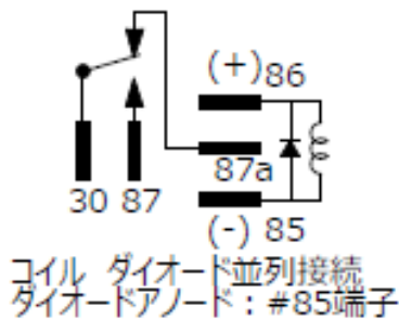
回路図①
