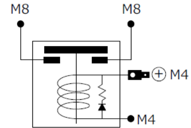
回路図③
