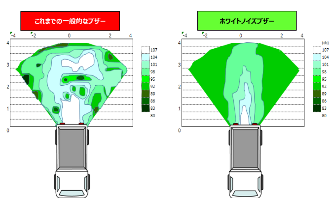
▲車両後方の音圧レベルマップ (イメージ)
