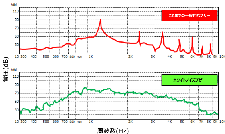
▲ブザーの周波数スペクトル (イメージ)
