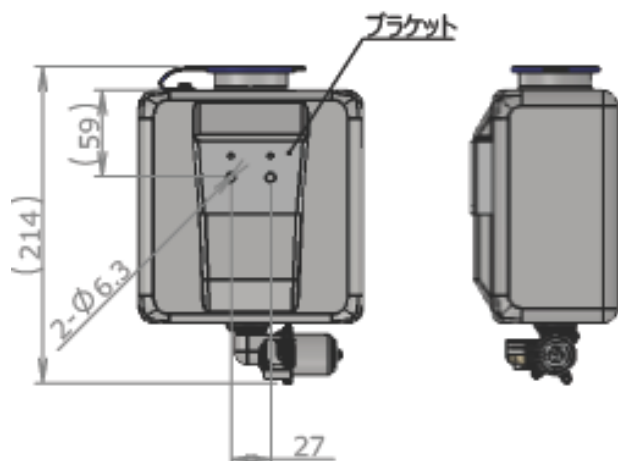
外観図⑦
